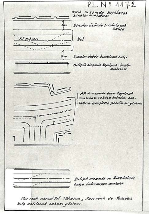
Yalova'daki yol tipleri (Taksim Atatürk Kitaplığı, HRT 7017/01)
