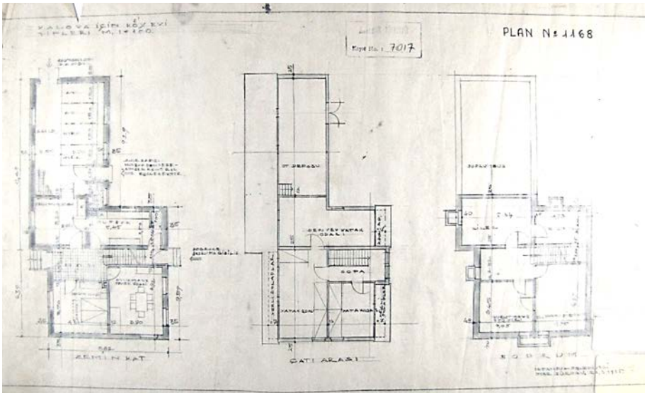
Yalova İçin Köy Evi Tipleri (Taksim Atatürk Kitaplığı, HRT 7017)
