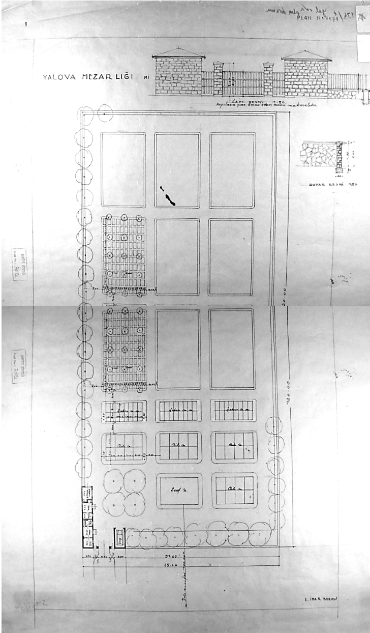
Yalova Mezarlığı Planı (Taksim Atatürk Kitaplığı, HRT 7021)
