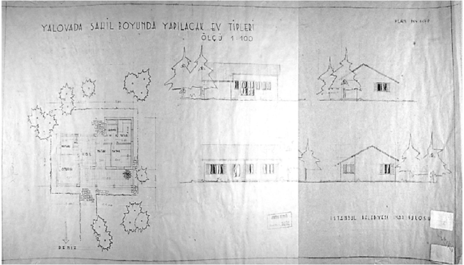
Yalova'da Sahil Boyunda Yapılacak Ev Tipleri (Taksim Atatürk Kitaplığı, HRT 7020)
